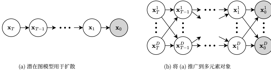
图1: 用于元素级扩散和多元素扩散的图模型图
